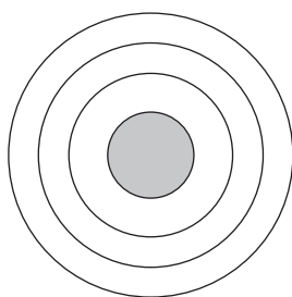
sodium atom
